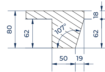
J-J (1:5)
