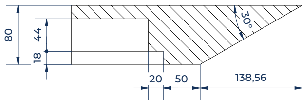
G-G (1:5)
